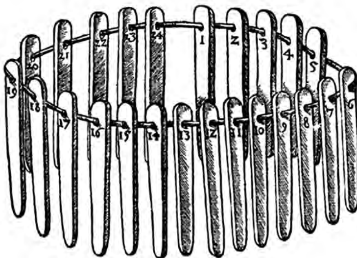
Puntas o juego de puntas para calcular el fino del oro y plata (las cifras del 1 al 24 son el número de las agujas o puntas a diferentes ligas).
